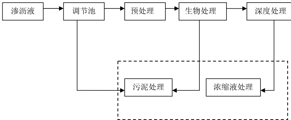
图 4.2.1 常规工艺流程
